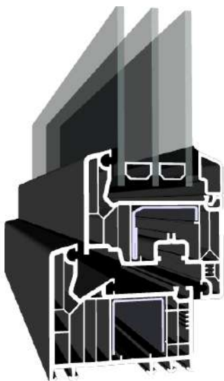
Normál ablak tok-szárny metszete
