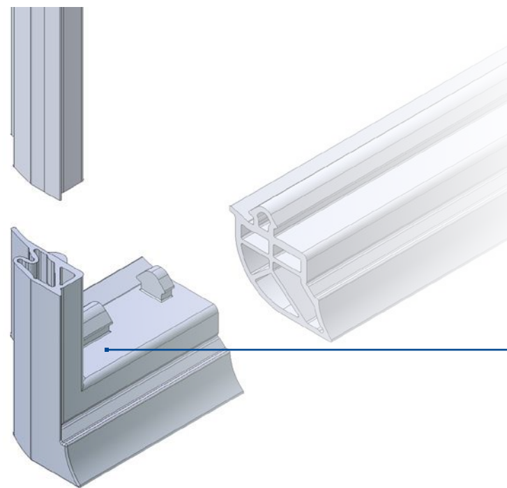
Vulkanizált sarokcsatlakozás Mindkét tömítést a gyártásban egy vulkanizált sarokon keresztül csatlakoztatják.
